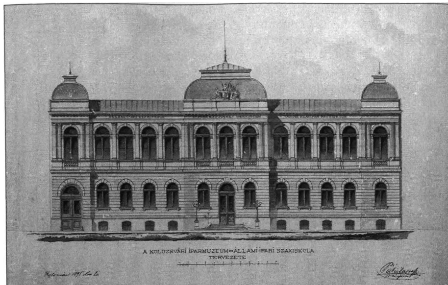
A Pákei Lajos által tervezett, 1896-1898 között felépült kolozsvári Erdélyrészi Technológiai Iparmúzeum (I. Ferenc József Technológiai Iparmúzeum) és az Építő-, Fa-, és Fémipari Iskola közös épületének főhomlokzata. Tervezet. 1895. november. MUEKvGyLt. Pákei-anyag, I-B-043. Reprodukció: Molnár Lehel
